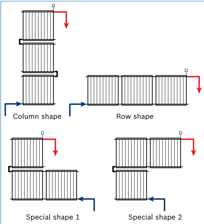
Example Solar-Lito Mini hydraulics schematics
