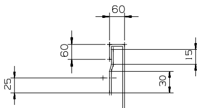
JOGGLE STRIP
