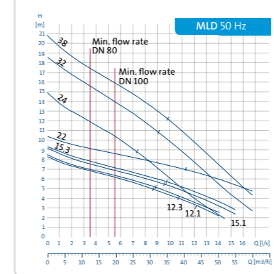
MULTILIFT MLD
